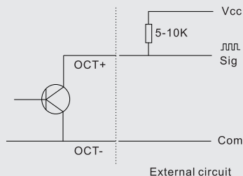
OCT 输出接线图
